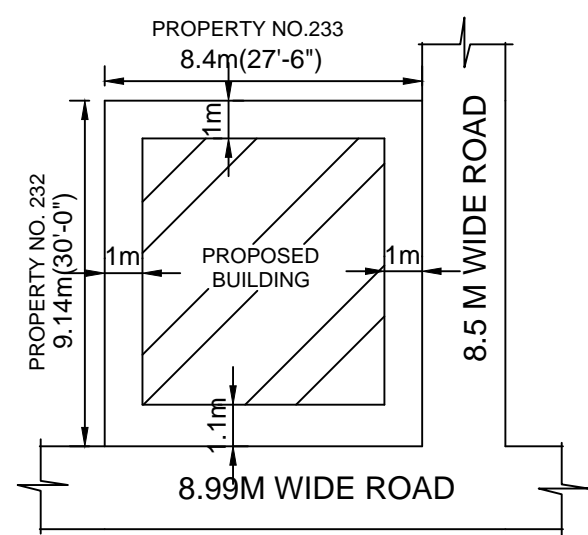
SITE PLAN(Scale 1:200)
